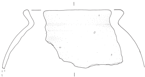
Abb. 1: Baltrum. Randscherbe eines Kugeltopfes aus dem 12. Jahrhundert vom Nordstrand der Insel Baltrum. M. 1:3. (Zeichnung: B. Kluczkowski)
