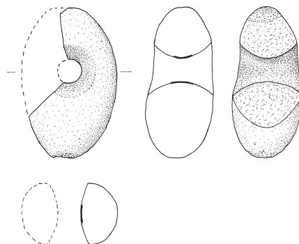
Abb. 1: Neermoor. Beschädigte Spitzhaue. (M. 1:3). (Zeichnung: B. Kluczkowski)
