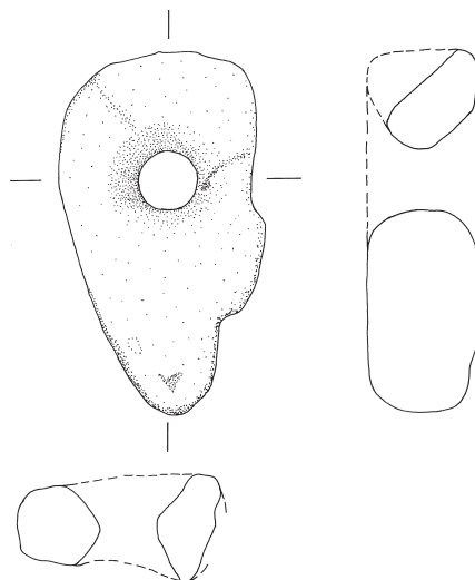
Abb. 1: Berumerfehn. An Nacken und Schneide beschädigte Spitzhaue. M. 1:3. (Zeichnung: G. Blumhoff)
