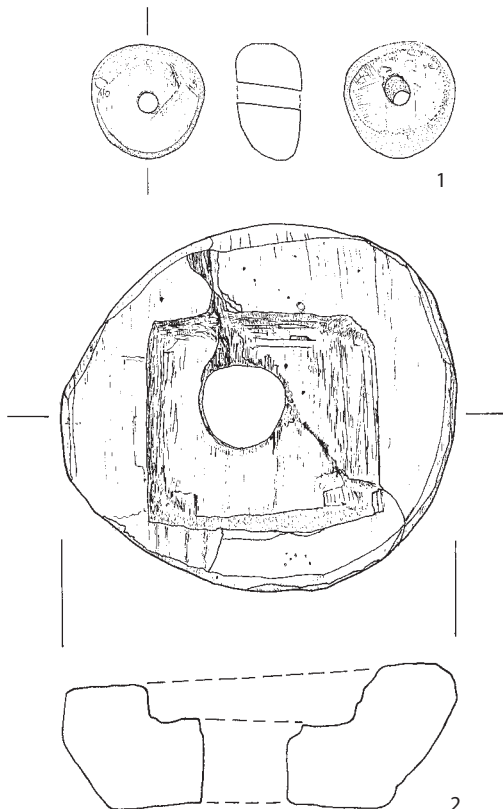
Abb. 1: Rahe. Funde aus einer Moorfläche nahe dem Upstalsboom-Hügel. 1 Bernsteinperle, 2 hölzernes Werkstück mit eckiger Ausnehmung und durchgängiger Lochung. M. 1:2. (Zeichnung: G. Kronsweide)
