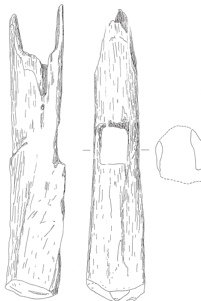
Abb. 2: Holtland. Pfostenstumpf mit Durchlochung. M. 1:12. (Zeichnung: G. Kronsweide)
