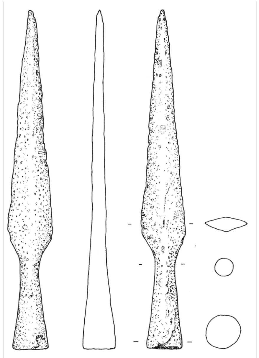
Abb. Holte (21). Eiserne Lanzenspitze mit kurzem, leicht dreieckigem Blatt. (Zeichnung: B. Kluczkowski)
